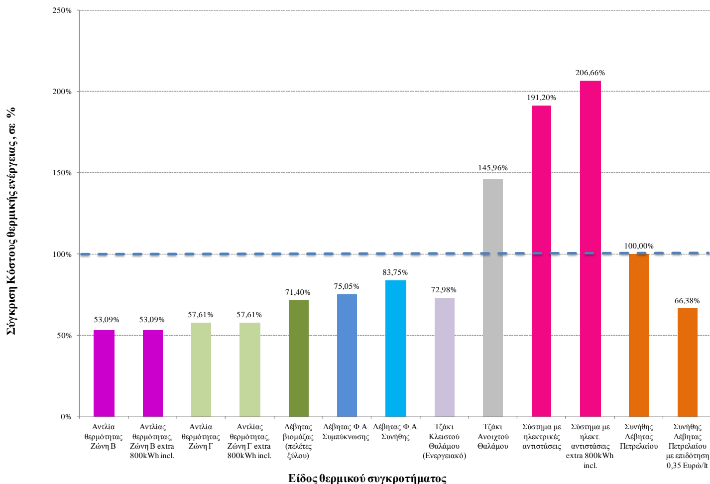
Διάγραμμα 2: Σύγκριση κόστους θερμικής ενέργειας σε %, σε σχέση με το κόστος ενός συγκροτήματος συνήθη λέβητα – καυστήρα πετρελαίου (για τιμή πετρελαίου ~1,041 €/lt), ανά είδος θερμικού συγκροτήματος
